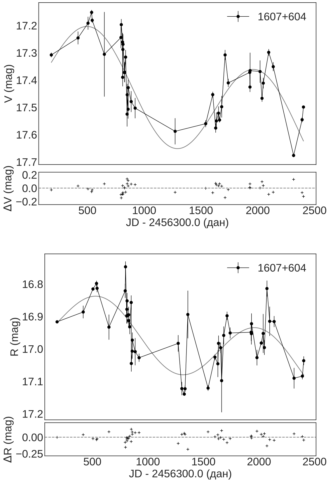
Слика 3.25: Криве сјаја објекта 1607+604 са функцијом усклађивања, коју чине линеарна функција и периодична; период износи 1464 дана у V (горе) и 1429 дана у R домену (доле).
