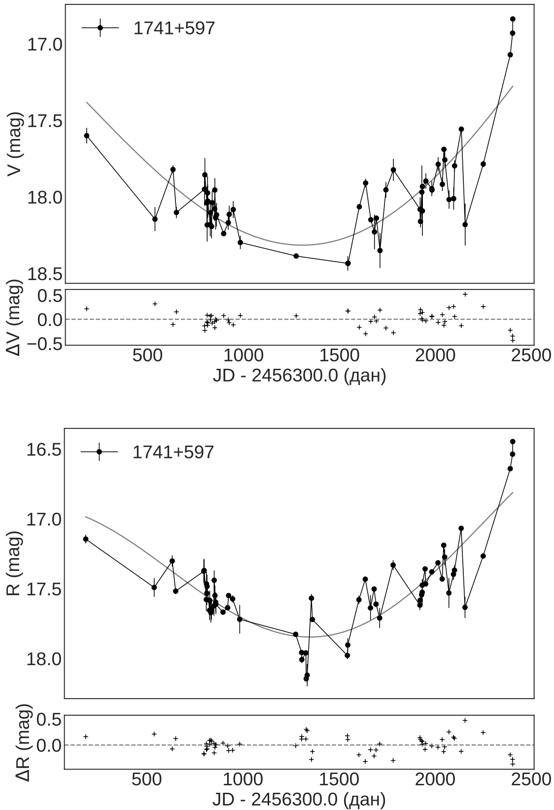
Слика 3.30: Криве сјаја објекта 1741+597 са функцијом усклађивања, коју чине линеарна функција и периодична; период износи 4987 дана у V (горе) и 3217 дана у R домену (доле).
