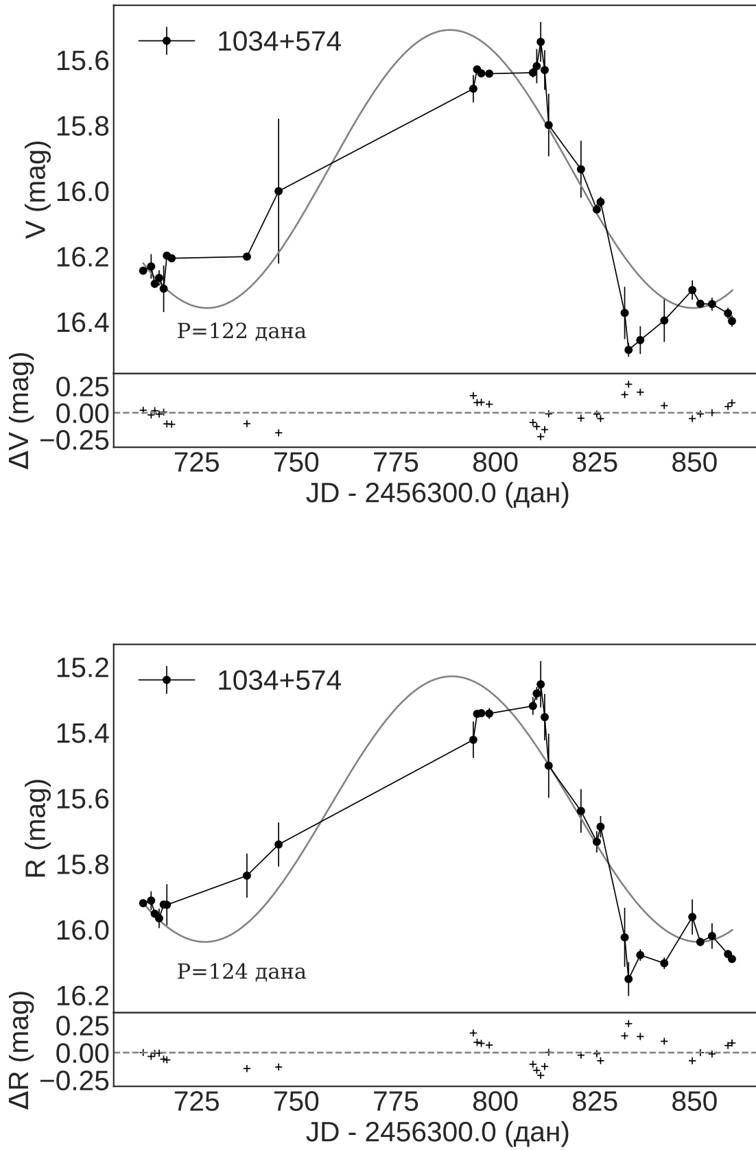
Слика 3.16: Криве сјаја објекта 1034+574 са функцијом усклађивања чији су параметри одређени методом DCDFT: у V домену (горе) и R домену (доле), само ТЈО посматрања. У доњем левом углу је вредност периода у данима.
