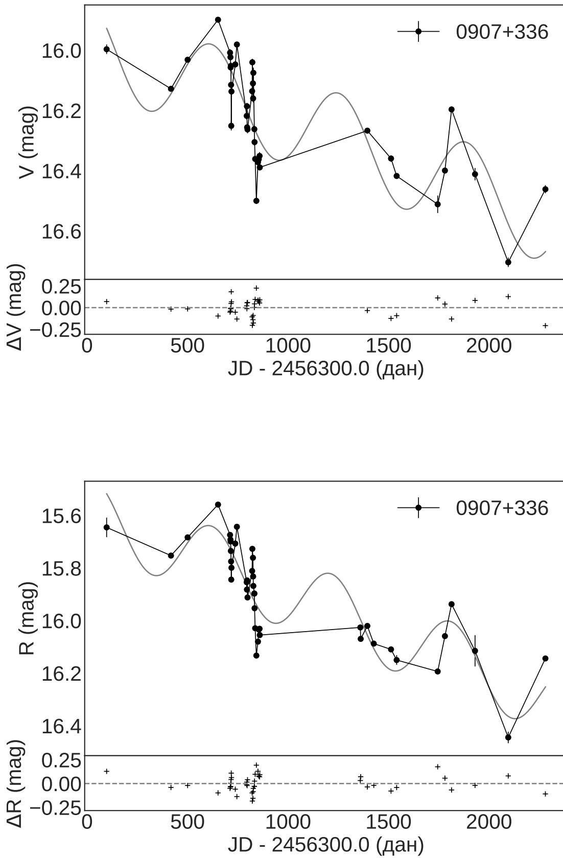
Слика 3.14: Криве сјаја објекта 0907+336 са функцијом усклађивања, коју чине линеарна функција и периодична са периодом од 634 дана у V (горе) и 595 дана у R домену (доле).
