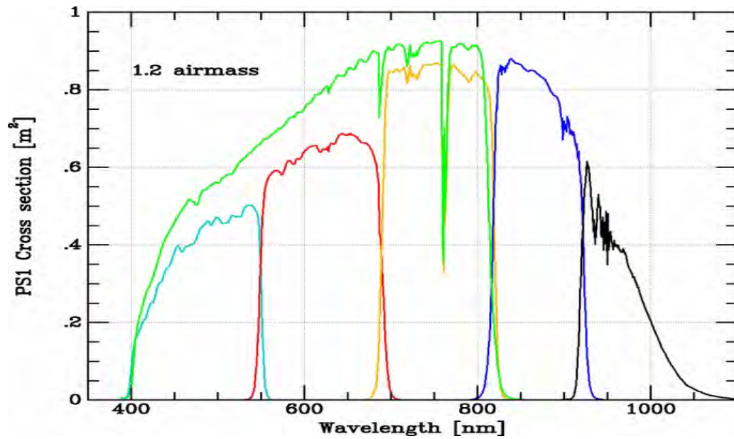
Слика 2.3: Шематски приказ Pan-STARRS фотометријског система g_{P1} (линија цијан боје), r_{P1} (црвена линија), i_{P1} (наранџаста), z_{P1} (плава), y_{P1} (црна) и w_{P1} (зелена), слика преузета из Tonry et al. (2012).
