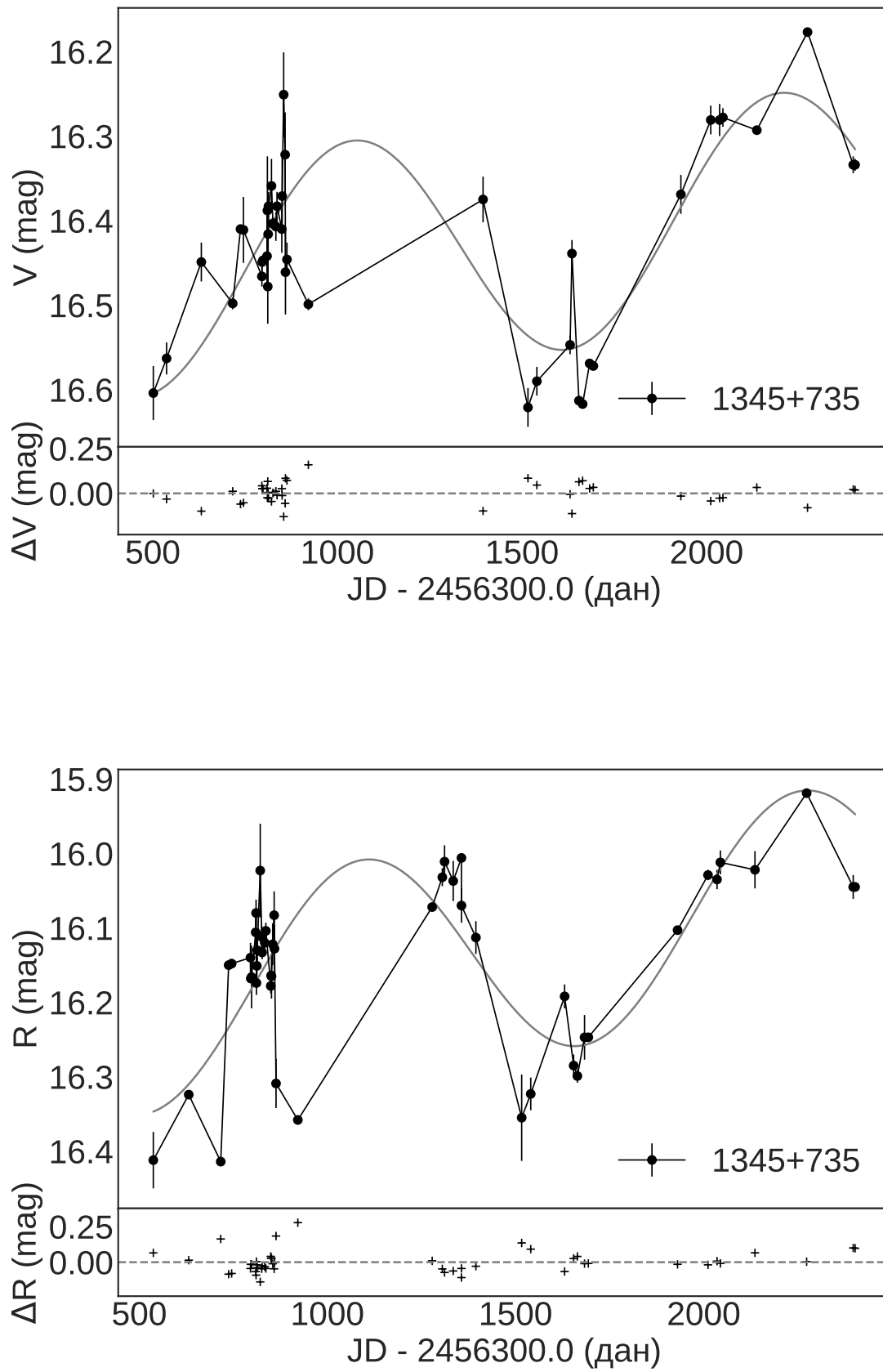
Слика 3.21: Криве сјаја објекта 1345+735 са функцијом усклађивања, коју чине линеарна функција и периодична; период износи 1156 дана у V (горе) и 1166 дана у R домену (доле).
