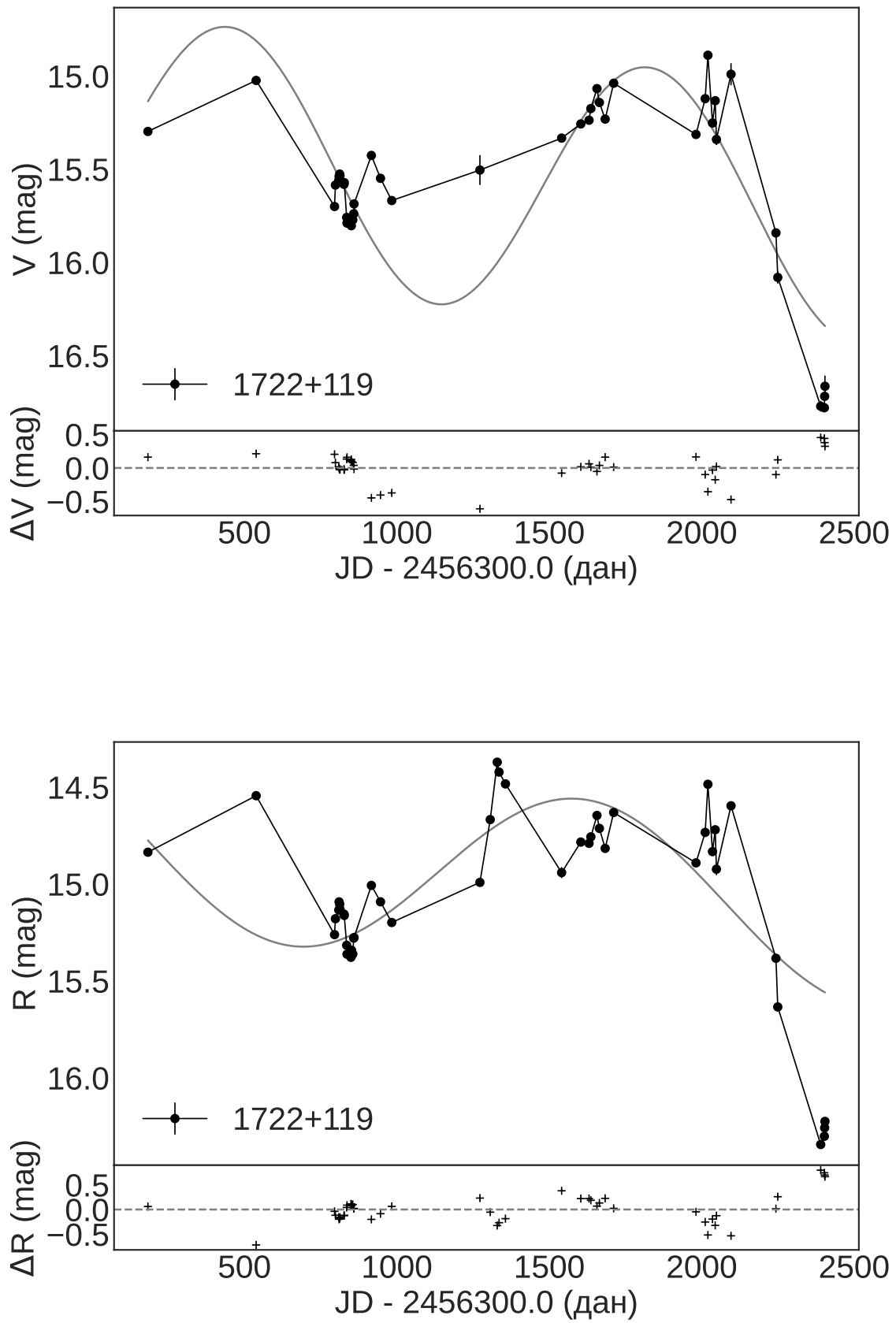
Слика 3.28: Криве сјаја објекта 1722+119 са функцијом усклађивања, коју чине линеарна функција и периодична; период износи 1377 дана у V (горе) и 1892 дана у R домену (доле).
