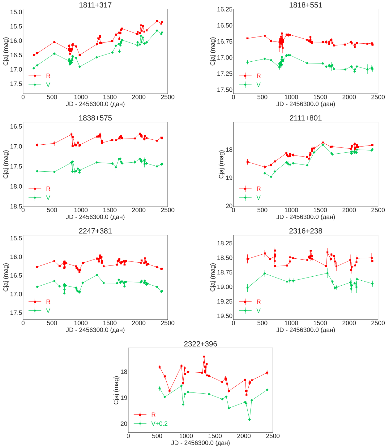
Слика В.1-5: Криве сјаја објеката 1811+317, 1818+551, 1838+575, 2111+801, 2247+381, 2316+238 и 2322+396.
