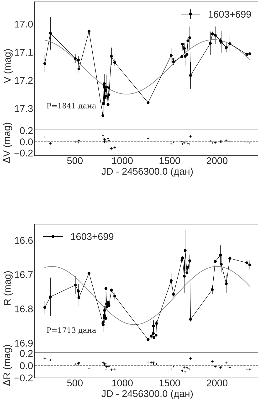
Слика 3.24: Криве сјаја објекта 1603+699 са функцијом усклађивања чији су параметри одређени методом DCDFIT: у V домену (горе) и R домену (доле). У доњем левом углу је вредност периода P .
