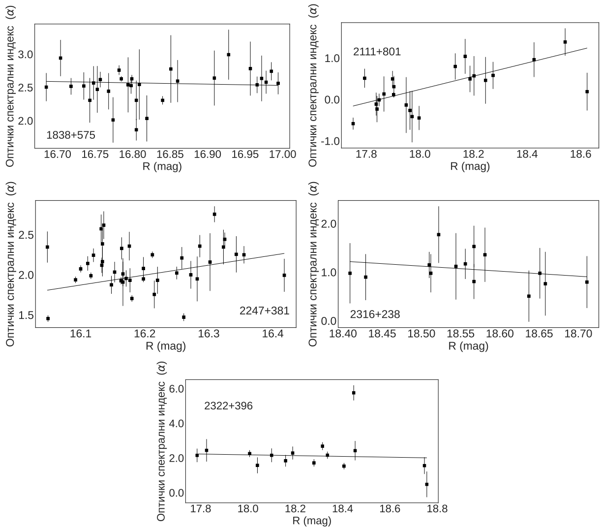
Слика Д.2-10: Зависност \alpha у односу на магнитуду R за објекте 1838+575, 2111+801, 2247+381, 2316+238 и 2322+396.
