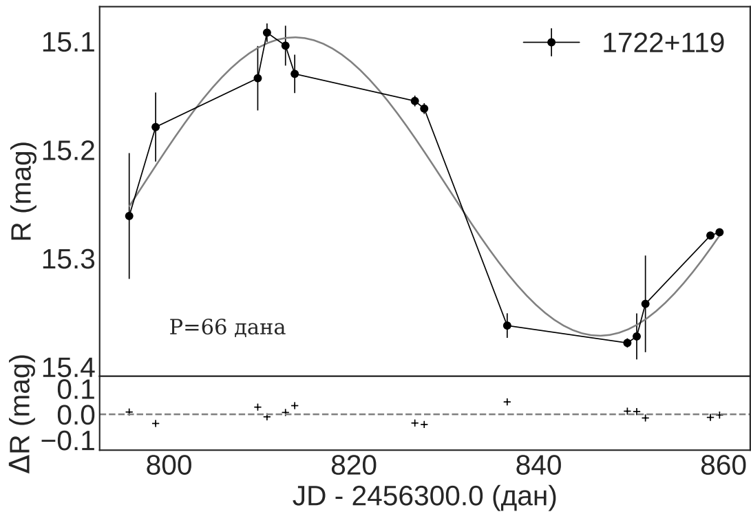
Слика 3.27: Криве сјаја објекта 1722+119 са функцијом усклађивања чији су параметри одређени методом DCDFT: у V домену (горе) и R домену (доле), само ТЈО посматрања. У доњем левом углу је вредност периода у данима.
