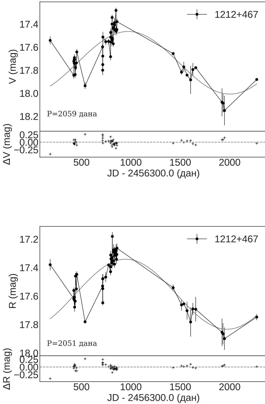
Слика 3.18: Криве сјаја објекта 1212+467 са функцијом усклађивања, чији су параметри одређени методом DCDFIT: у V домену (горе) и R домену (доле). У доњем левом углу је вредност периода P .
