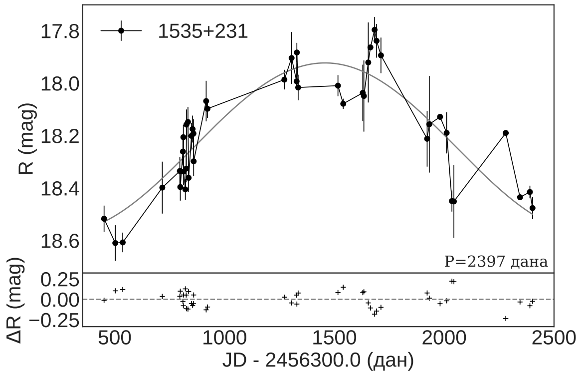
Слика 3.23: Криве сјаја објекта 1535+231 са функцијом усклађивања чији су параметри одређени методом DCDFT: у V домену (горе) и R домену (доле). У доњем десном углу је вредност периода P .
