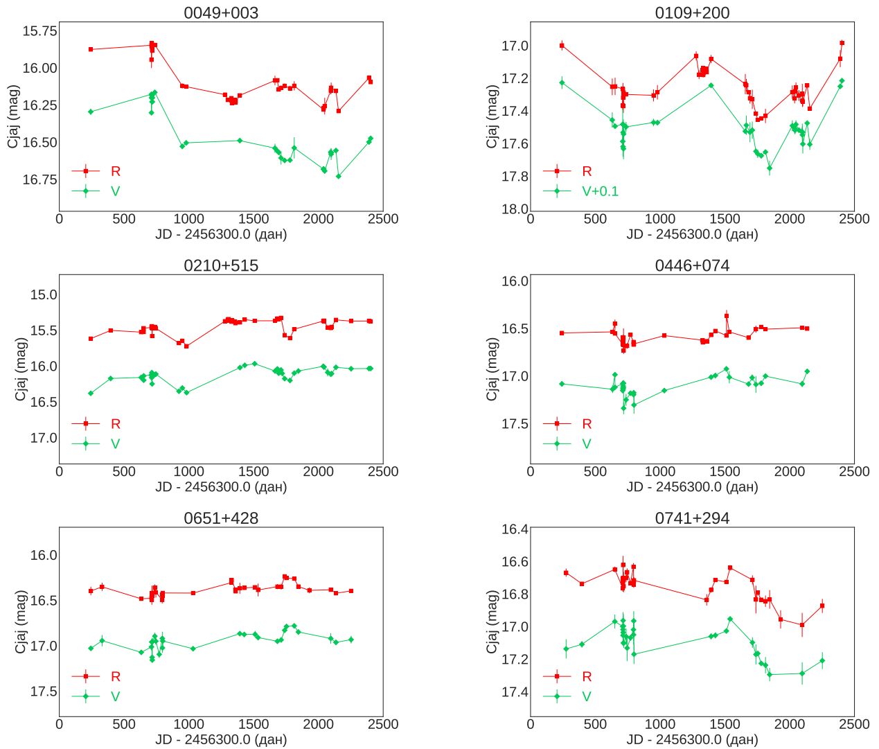
Слика В.1-1: Криве сјаја објекта 0049+003, 0109+200, 0210+515, 0446+074, 0651+428 и 0741+294.
