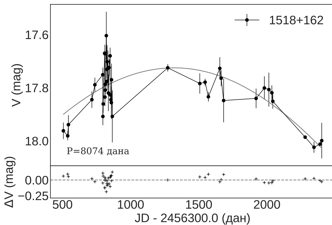
Слика 3.22: Крива сјаја објекта 1518+162 у V домену са функцијом усклађивања чији су параметри одређени методом DCDFIT. У доњем левом углу је вредност периода P .
