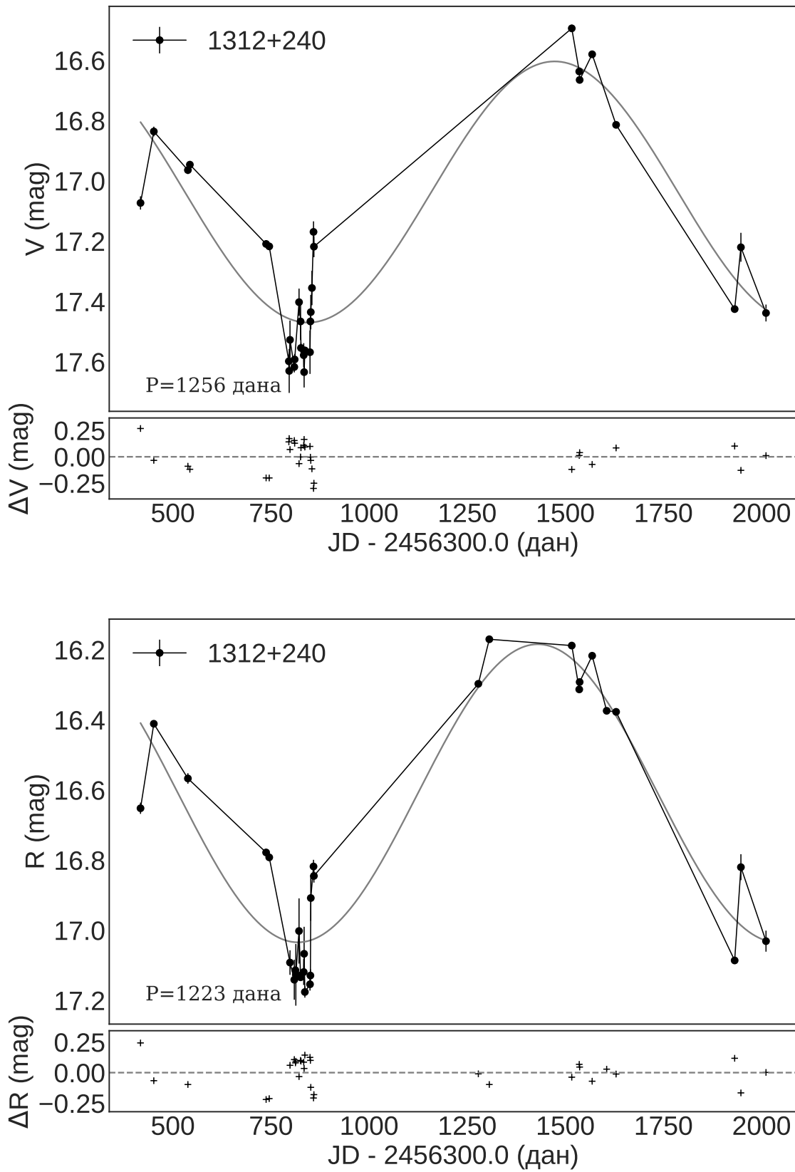
Слика 3.20: Криве сјаја објекта 1312+240 са функцијом усклађивања чији су параметри одређени методом DCDFT: у V домену (горе) и R домену (доле). У доњем левом углу је вредност периода у данима.
