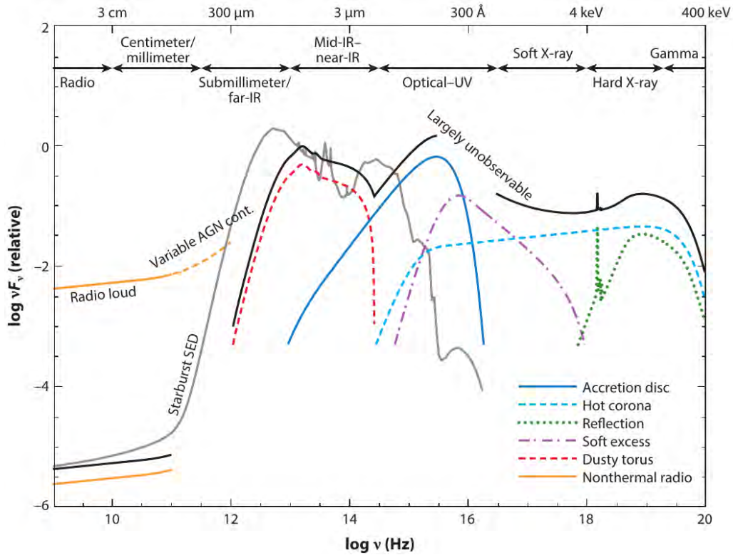
Слика 1.3: Шематски приказ спектралне расподеле енергије АГЈ заснованог на посматраном SED радио-слабих АГЈ, слика је преузета из Hickox & Alexander (2018) и представља адаптацију слике из Harrison (2014).
