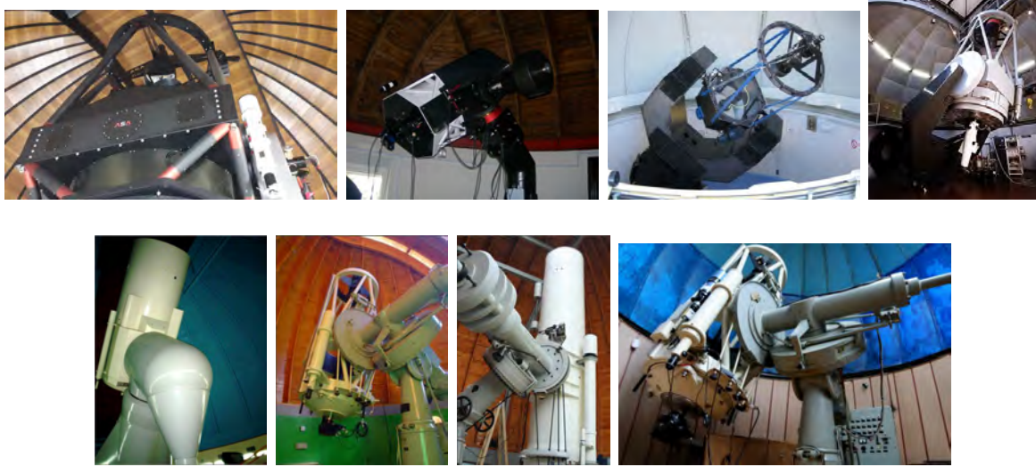
Слика 2.1: Фотографије телескопа. Горњи ред (са лева на десно): АСВ 1.4 m, АСВ 60 cm*, ТЈО 80 cm**, LFOA 1.5 m***. Доњи ред: Рожен 2 m*, 60 cm*, 50/70 cm* и Белоградчик 60 cm*. Аутори фотографија: АСВ 1.4 m Миљана Јовановић, LFOA проф. Franz Kerschbaum, Рожен телескопа др Д. Колев и П. Маркишки и Белоградчик П. Маркишки. * Сlike су преузете са званичних сајтова поменутих опсерваторија, ** преузета из билтена Катедре за физику и нуклерано инжењерство Политехничког Универзитета у Каталонији, *** преузета са Wikipedia странице опсерваторије.
