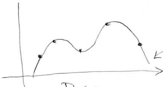
P_n(x)
