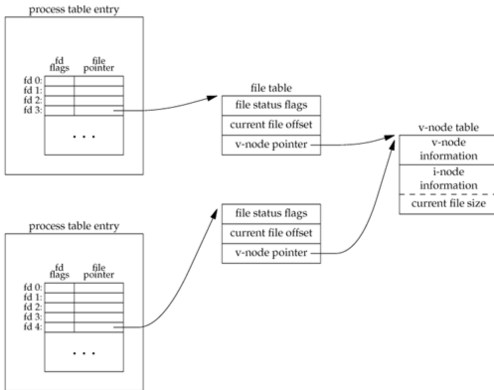
Dva procesa koji imaju isti fajl otvoren
