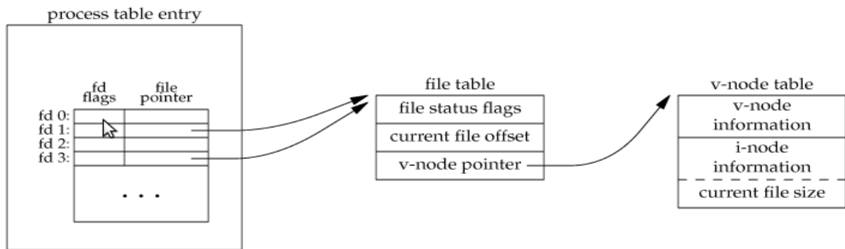
Kernel strukture podatak nakon izvršavanja dup(1)
