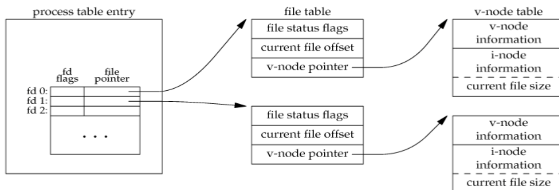
Kernel strukture podataka za otvorene fajlove
